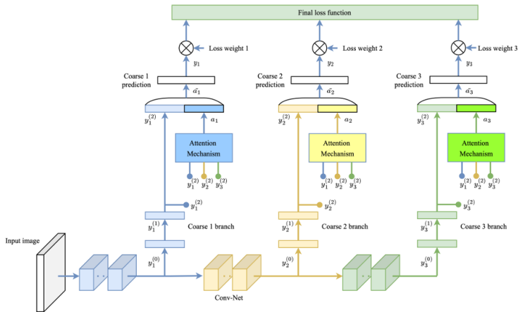
Figura: Arquitetura BA-CNN
