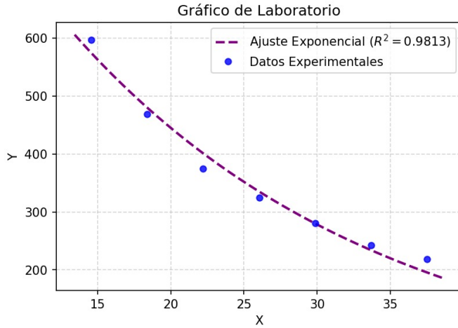
Fig. 8. Gráfico original de la Tabla VI. El eje X representa la longitud efectiva L' en cm y el eje Y la frecuencia f en Hz. El ajuste exponencial mostrado ( R^2 = 0.9813 ) es descriptivo; el modelo físico es f = v/(4L') .
