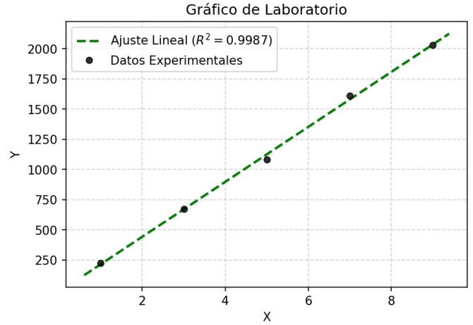
Fig. 7. Gráfico original de la Tabla III. El eje X representa el armónico asignado n y el eje Y la frecuencia f_n en Hz. Ajuste lineal: R^2 = 0.9987 .
