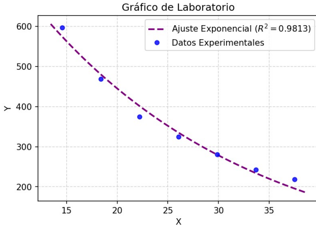
Fig. 8. Gráfico de la Tabla VI. El eje X representa la longitud efectiva L' en cm y el eje Y la frecuencia f en Hz. El ajuste exponencial mostrado ( R^2 = 0.9813 ) es descriptivo; el modelo físico es f = v/(4L') .
