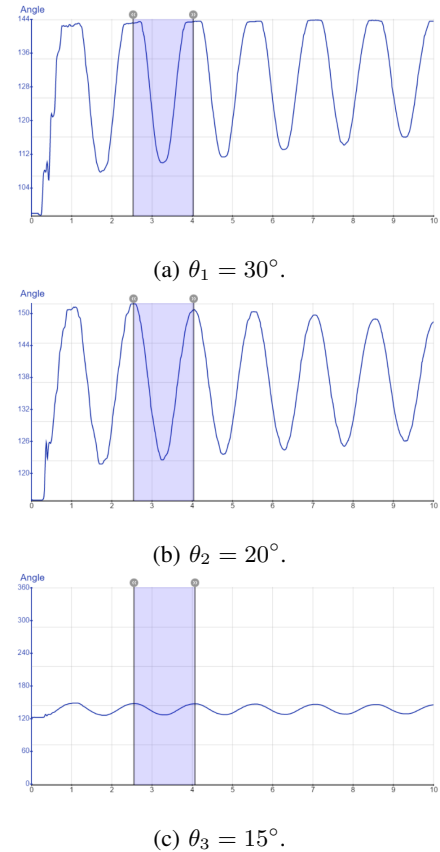
Fig. 3: Registros experimentales de la posición angular en función del tiempo para tres amplitudes iniciales diferentes.
