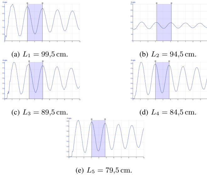
Fig. 2: Curvas experimentales de posición angular versus tiempo obtenidas al modificar la longitud del péndulo.
