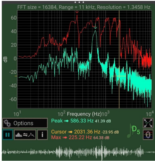
Fig. 6. Espectro registrado con un máximo de 225.22 Hz, FFT de 16384 puntos y resolución de 1.3458 Hz. Los niveles mostrados son indicadores de la aplicación.
