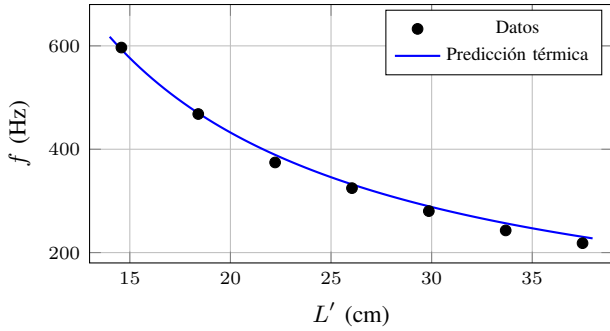
Fig. 8. Frecuencia frente a longitud efectiva. La curva es la predicción térmica f = v_T / (4L') , con v_T = 345.875 m/s, para el modelo de tubo cerrado.
