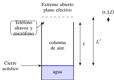
Fig. 4. Geometría acústica esquemática: \ell es la longitud física y L' = \ell + 0.3D la efectiva. La ubicación del teléfono es esquemática. No está a escala.
