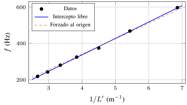
Fig. 9. Frecuencia frente a longitud inversa: ajuste libre f = (90.3164 \text{ m/s})x - 24.2152 \text{ Hz} , R^2 = 0.999284 . La línea discontinua muestra el ajuste forzado al origen como contraste.
