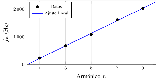
Fig. 7. Frecuencia frente a armónico asignado: f_n = (227.539 \text{ Hz})n - 13.017 \text{ Hz} , R^2 = 0.998668 .
