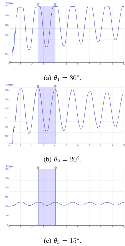
Fig. 5: Registros experimentales de la posición angular en función del tiempo para tres amplitudes iniciales diferentes.
