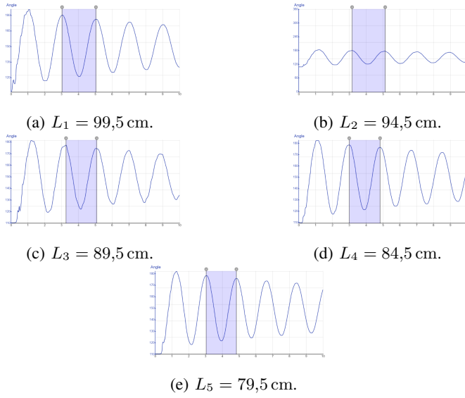
Fig. 4: Curvas experimentales de posición angular versus tiempo obtenidas al modificar la longitud del péndulo.
