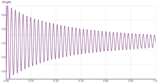
Fig. 6: Registro continuo de decaimiento temporal en el régimen subamortiguado.
