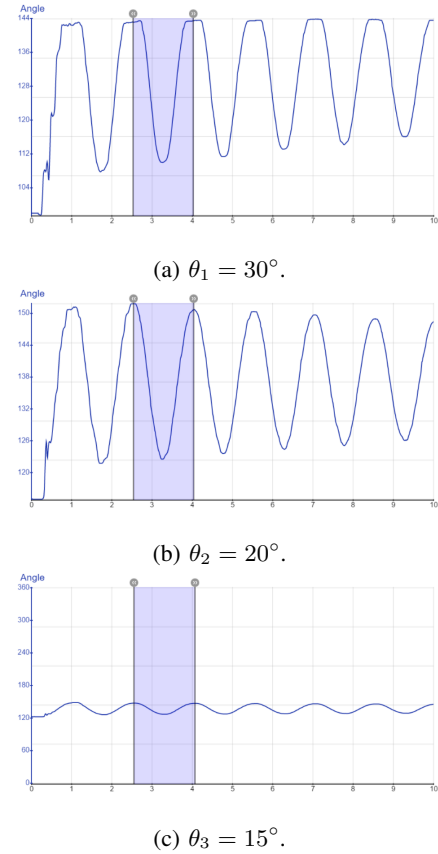
Fig. 6: Registros experimentales de la posición angular en función del tiempo para tres amplitudes iniciales diferentes.
