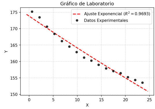
Fig. 8: Curva de regresión y ajuste del modelo para la envolvente exponencial.
