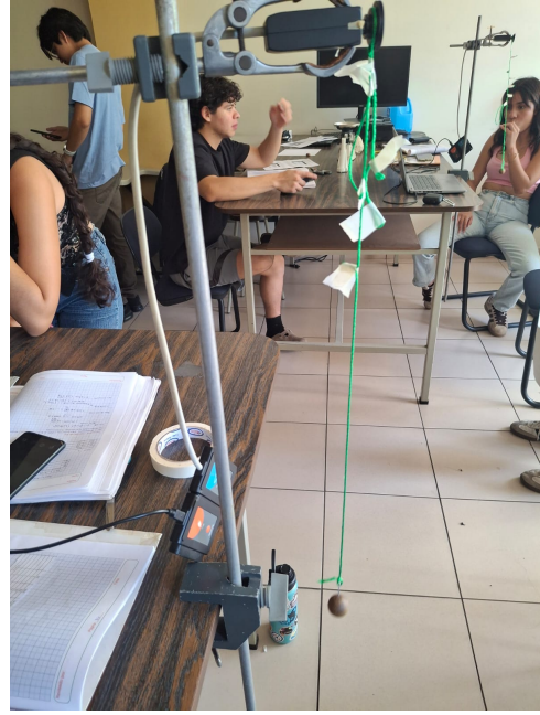
Fig. 1: Montaje experimental utilizado para el estudio del péndulo simple. Se observa el sensor de rotación NeuLog, el cordel y la esfera suspendida del sistema.
