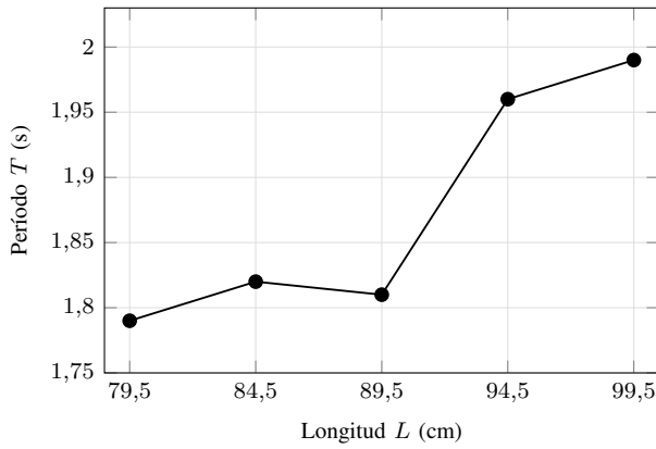
Fig. 4: Período experimental T en función de la longitud L del péndulo.
