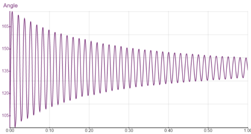
Fig. 7: Registro continuo de decaimiento temporal en el régimen subamortiguado.
