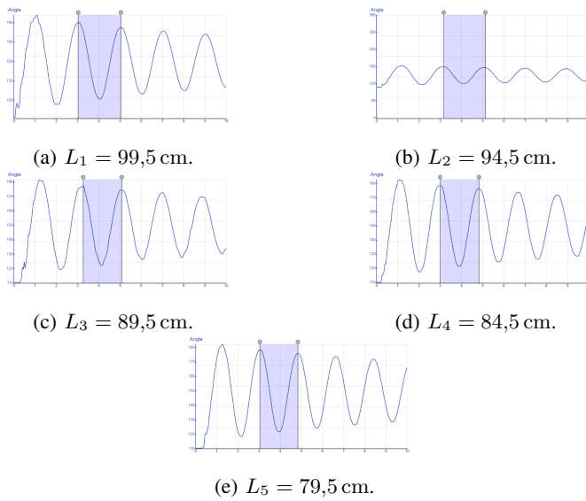
Fig. 5: Curvas experimentales de posición angular versus tiempo obtenidas al modificar la longitud del péndulo.
