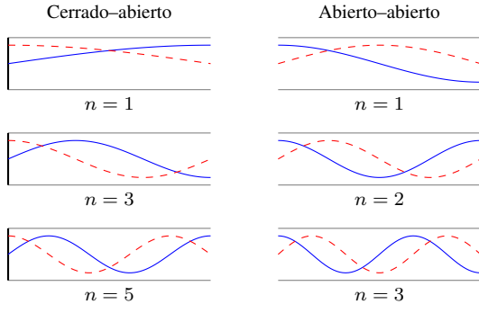
Fig. 1. Perfiles espaciales normalizados de desplazamiento (línea continua) y presión (discontinua), en un instante representativo. Tubo cerrado-abierto: n = 1, 3, 5 ; abierto-abierto: n = 1, 2, 3 . Se representan modos ideales, no mediciones.
