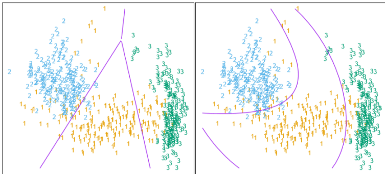
Figura 1: A la izquierda el clasificador \mathbf{x} y la derecha el clasificador \tilde{\mathbf{x}} . Fuente Hastie et al. (2008)
