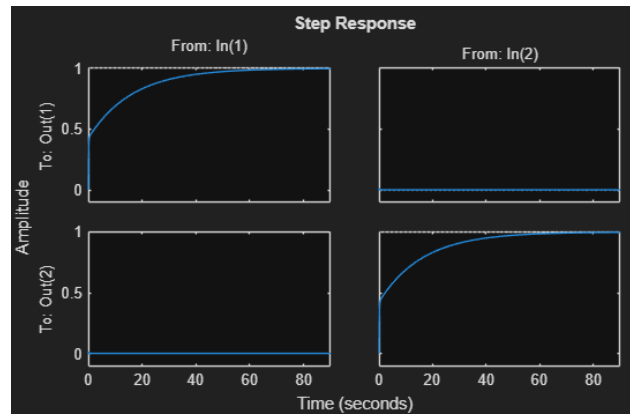
Figura 4: CRegolazione delle realizzazioni del sistema nominale ad anello chiuso
