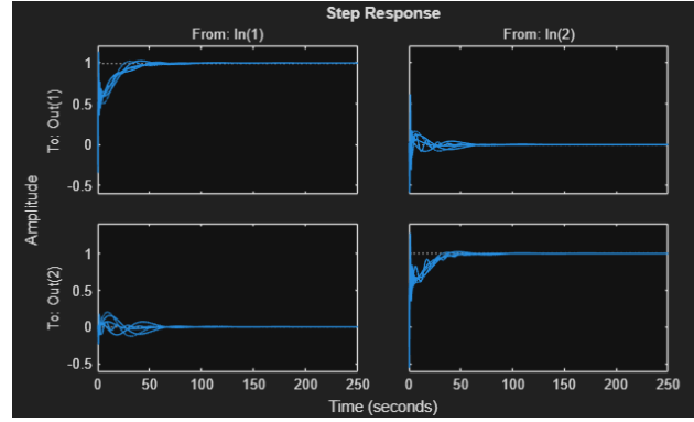
Figura 5: CRegolazione delle realizzazioni del sistema con incertezza ad anello chiuso per \omega_0 = 0.1236
