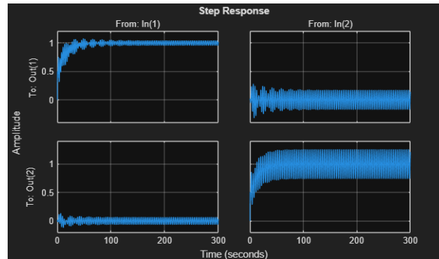
Figura 6: CRegolazione delle realizzazioni del sistema con incertezza ad anello chiuso- worst case
