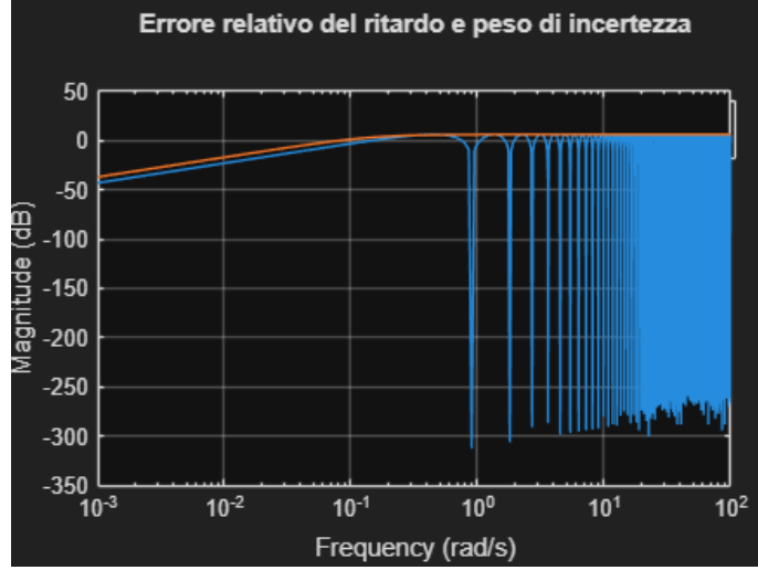
Figura 1: Confronto tra l'errore relativo dovuto al ritardo e il peso di incertezza.
