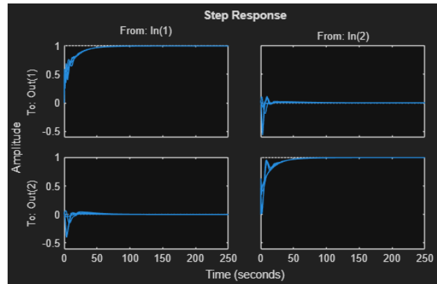
Figura 3: Regolazione delle realizzazioni del sistema ad anello chiuso con incertezza
