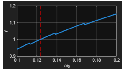
Figura 2: Limite \omega_0 - gamma
