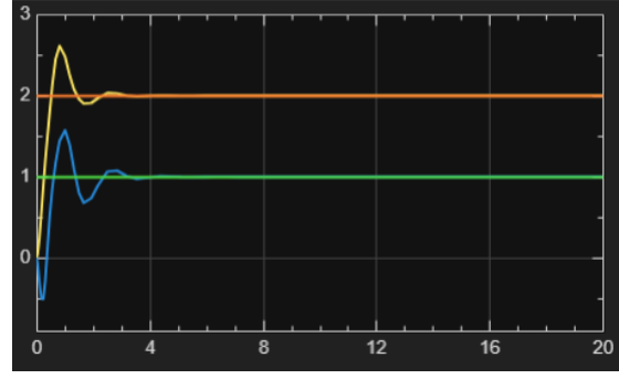
(b) Risposta con T_s = 1\text{ s} e \zeta = 0.4
