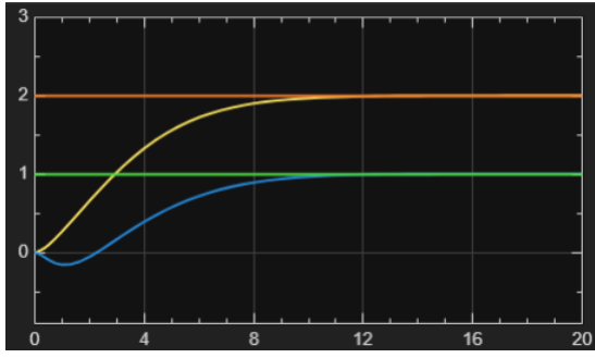
(a) Risposta con T_s = 3\text{ s} e \zeta = 1
