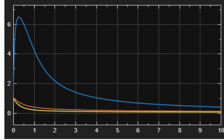
Figura 19: Andamento delle velocità angolari del sistema sottoattuato durante la fase di stabilizzazione.
