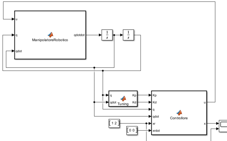
Figura 30: Schema Simulink del controllore nello spazio operativo con blocco di tuning basato sulla massa operativa \Delta .
