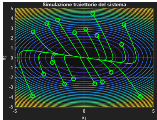
Figura 8: Simulazione Matlab delle traiettorie tramite ginput
