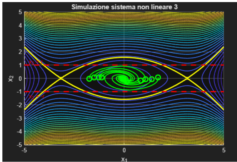
Figura 11: Simulazione Matlab delle traiettorie tramite ginput
