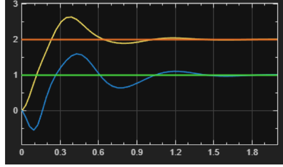
(b) Risposta con T_s = 1 s e \zeta = 0.4
