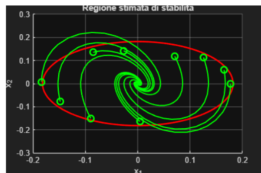
(b) Traiettorie per diverse x_0
