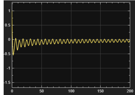
Figura 22: Andamento della prima componente dell'errore di tracking nel caso di controllo adattativo.
