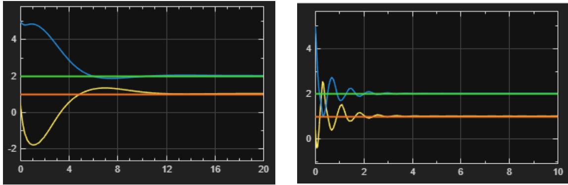
Caso 1: \xi = 0.7 , T_s = 3 s
