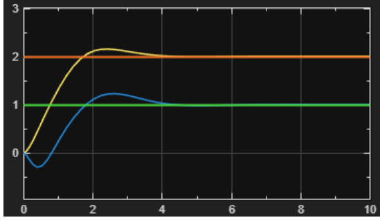
(a) Risposta con T_s = 3 s e \zeta = 1
