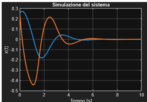
(a) Simulazione con x(0) = (0.25, 0.25) .
