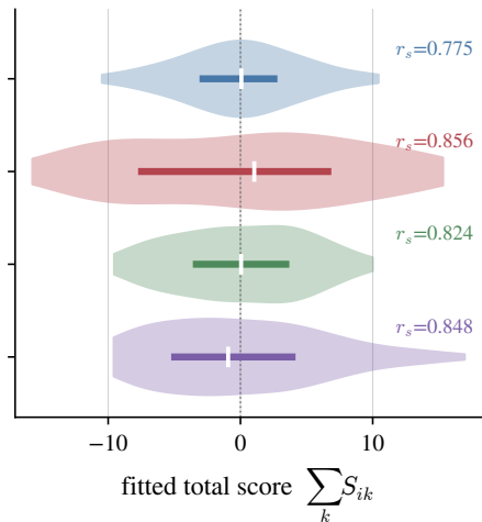
ASAP
