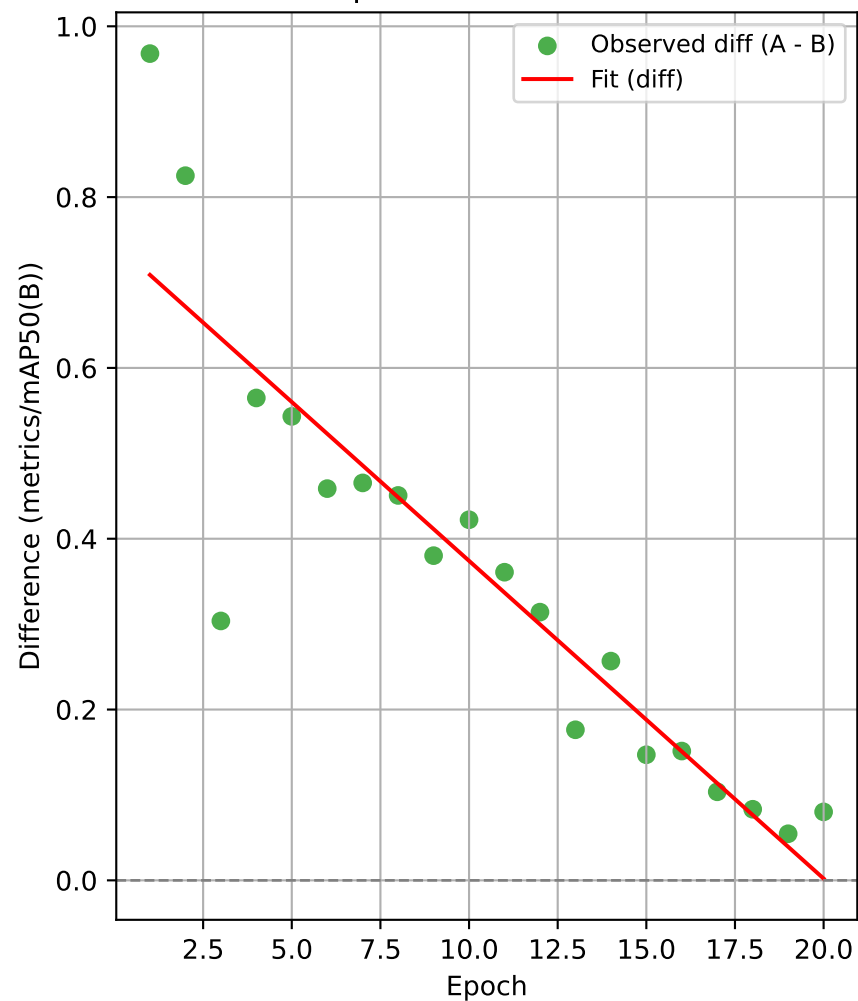
YOLO – UnpretrainedYOLO : difference
