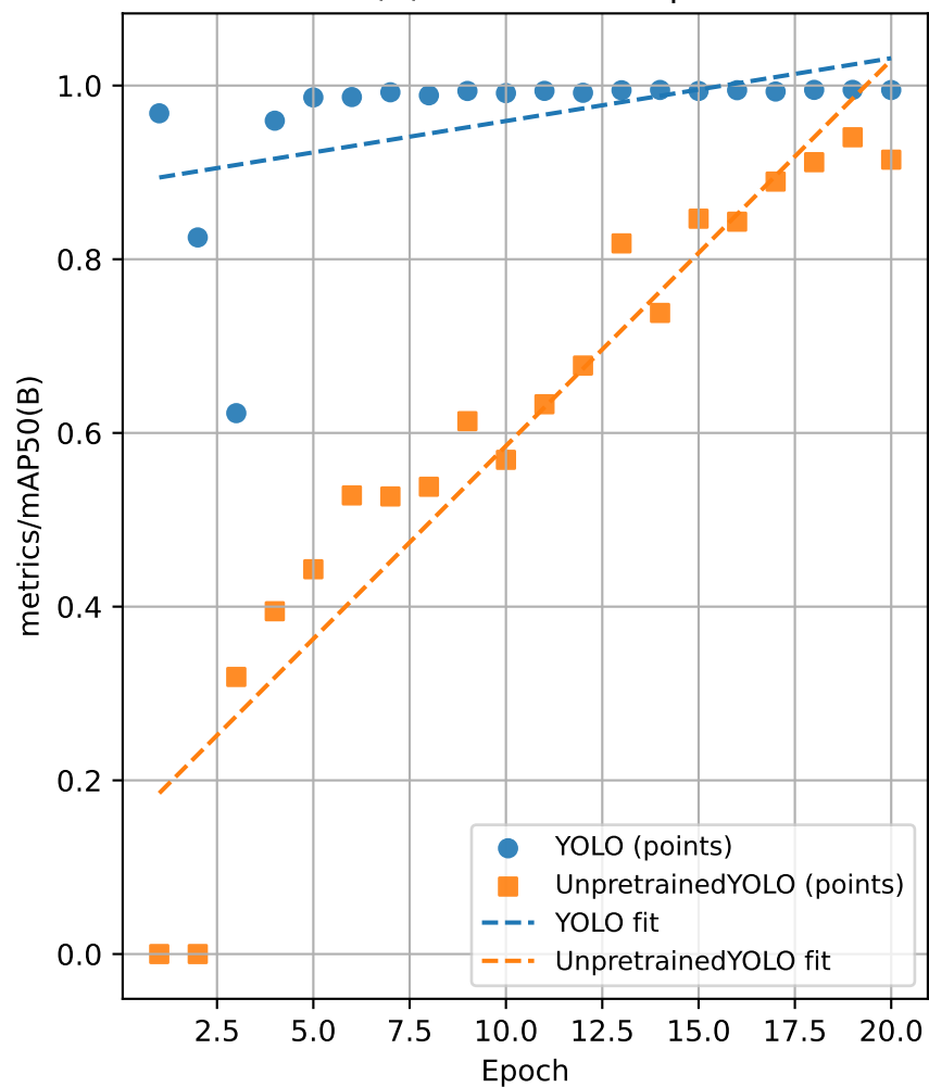
metrics/mAP50(B) — YOLO & UnpretrainedYOLO
