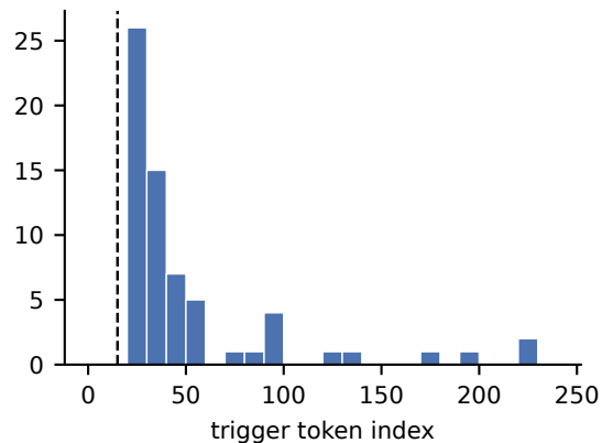
Mistral GSM8K Sinkhorn (n=65)
