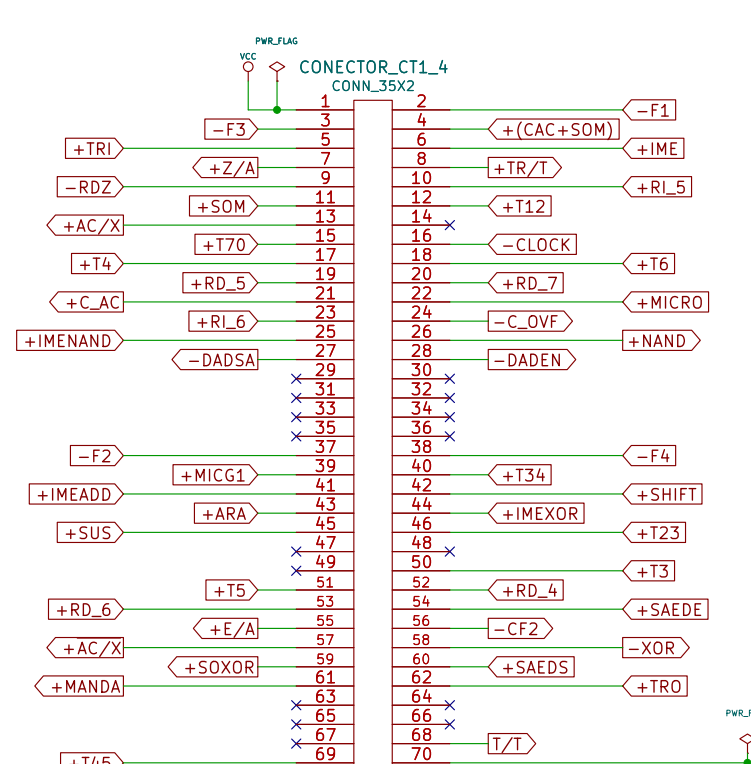
Placa CT1-4: Sinais de controle.
