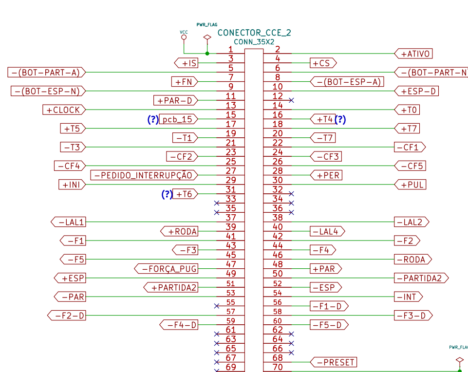
Placa CCE-2: Control de estado.
