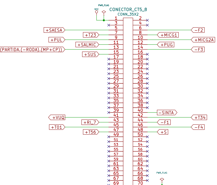
Placa CT5-8: Sinais de controle
