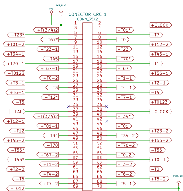
Placa CRC-1: Relógio central.
