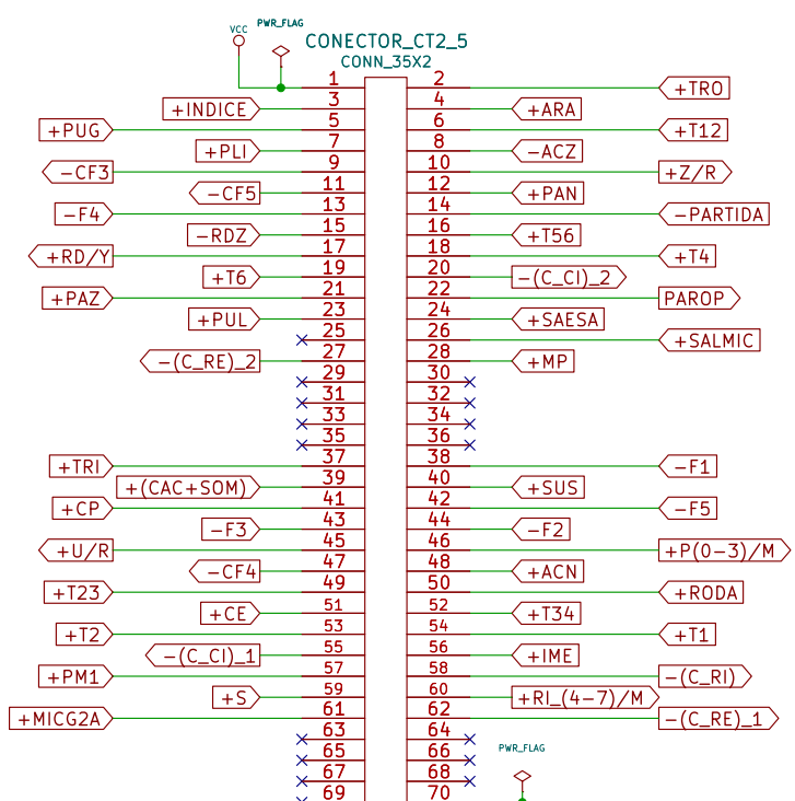
Placa CT2-5: Sinais de controle.
