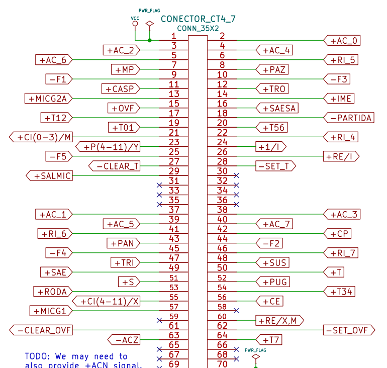
Placa CT4-7: Sinais de controle
