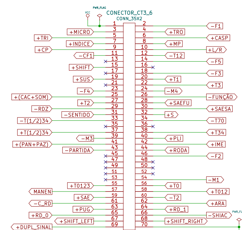
Placa CT3-6: Sinais de controle
