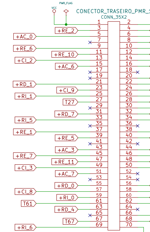
CONECTOR TRASEIRO PMR-1: PLACA MOSTRA REGISTRADORES Drivers para os LEDs.
