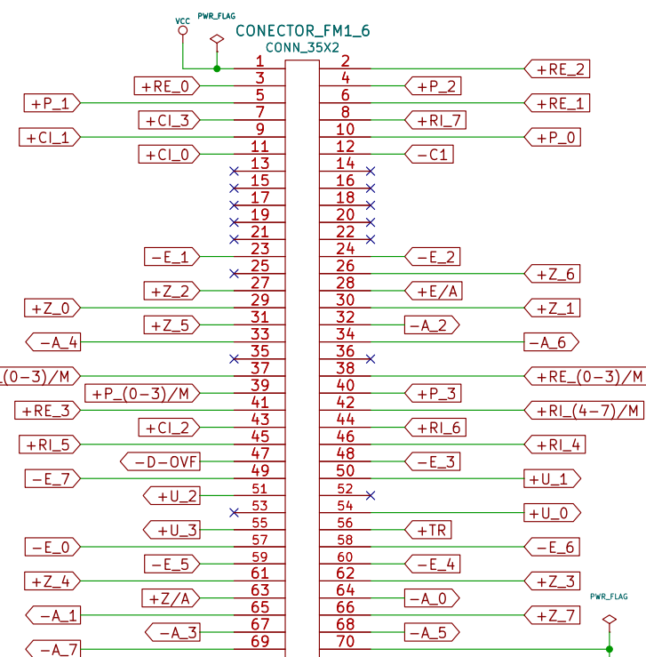
Placa FM1-6: Mais-um e porta de seleção 6
