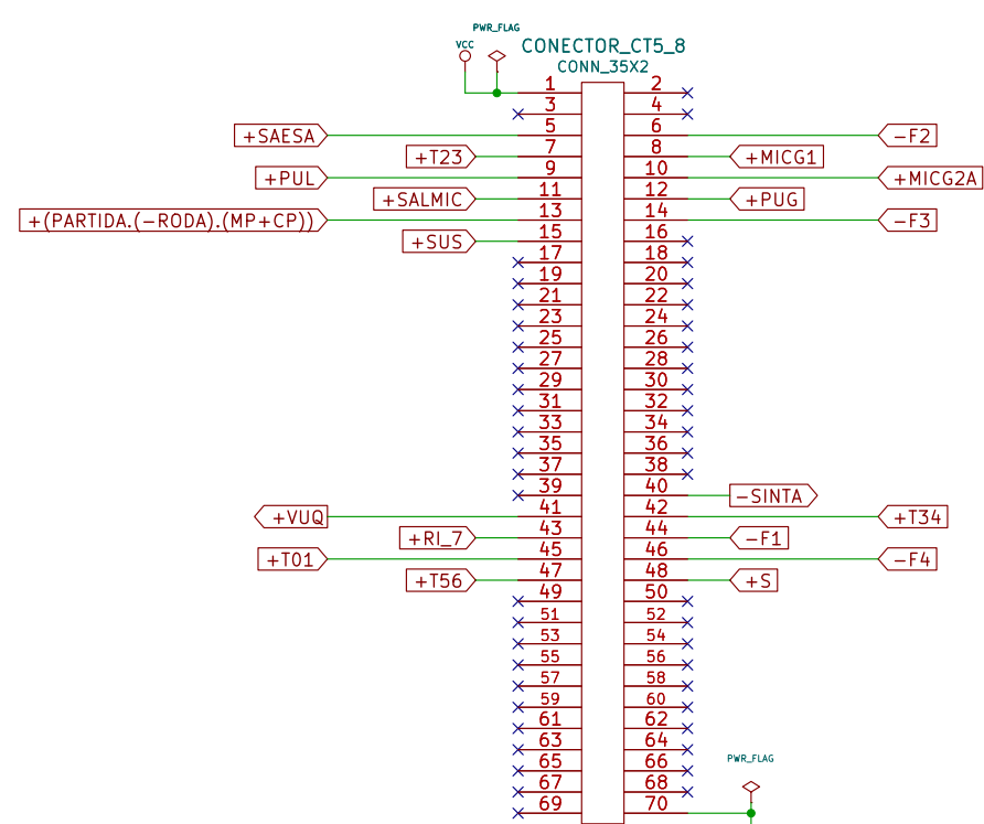
Placa CT5-8: Sinais de controle
