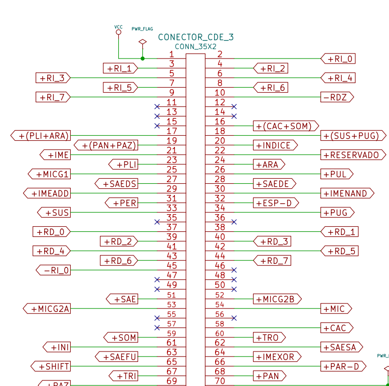
Placa CDE-3: Decodificador de instruções.
