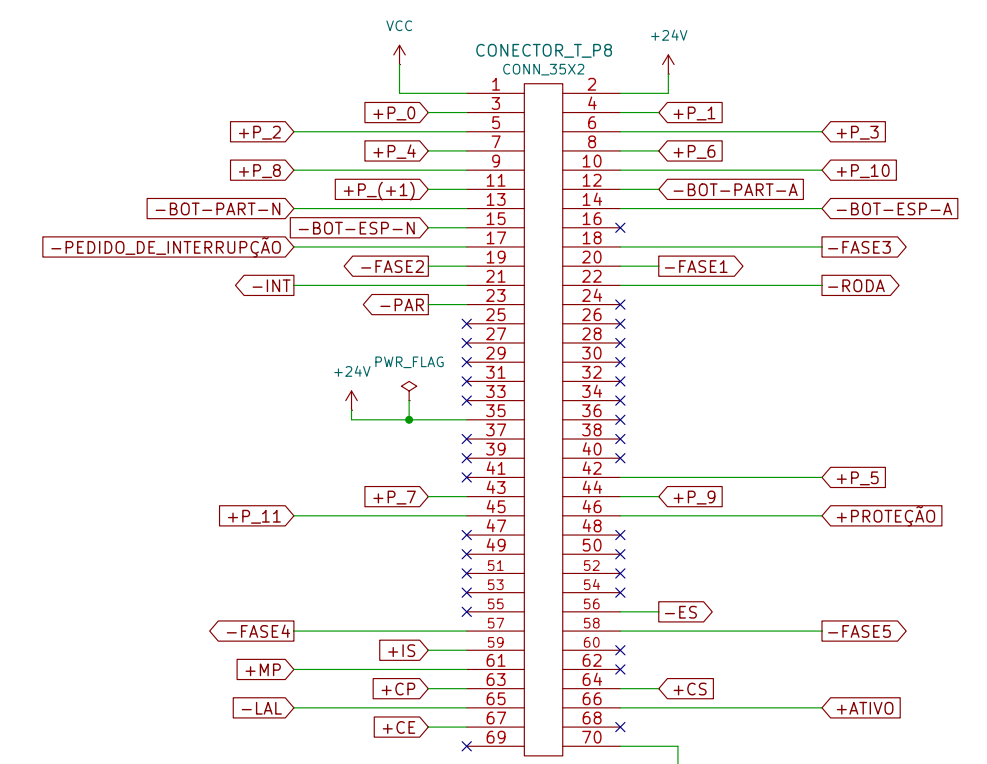
CONECTOR TRASEIRO
