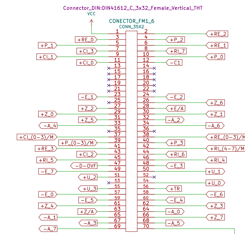
Placa FML-6: Mais um a porta de seleção 6.
