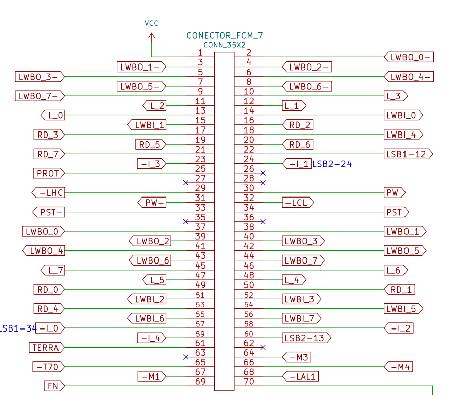
Placa FCM-7: Interface com memória.
