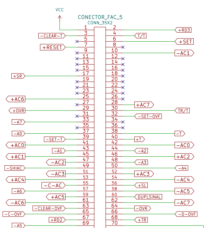
Placa FAC-5: Acumulador.
