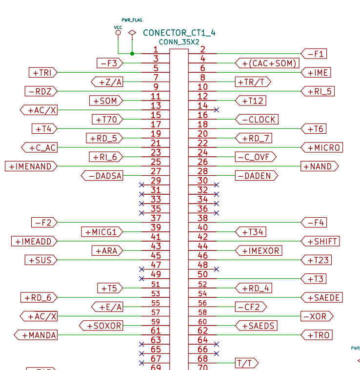
Placa CT1-4: Sinais de controle.
