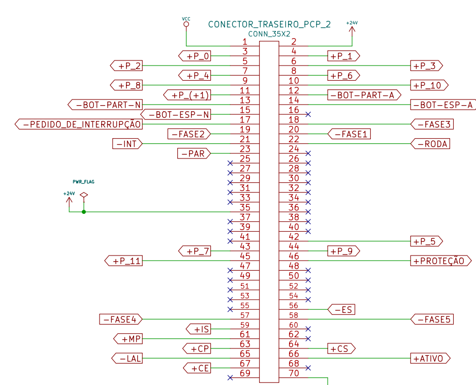
PCP-2: PLACA CHAVES E PILOTO "Debounce" para chaves e drivers para lâmpadas piloto.
