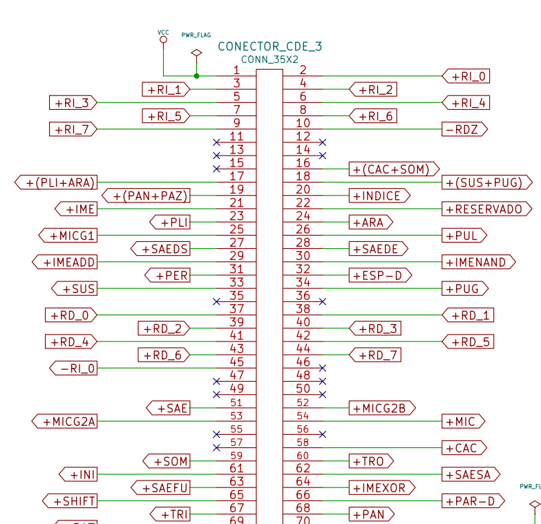
Placa CDE-3: Decodificador de instruções
