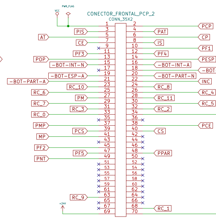
PCP-2: PLACA CHAVES E PILOTO "Debounce" para chaves e drivers para lâmpadas piloto.
