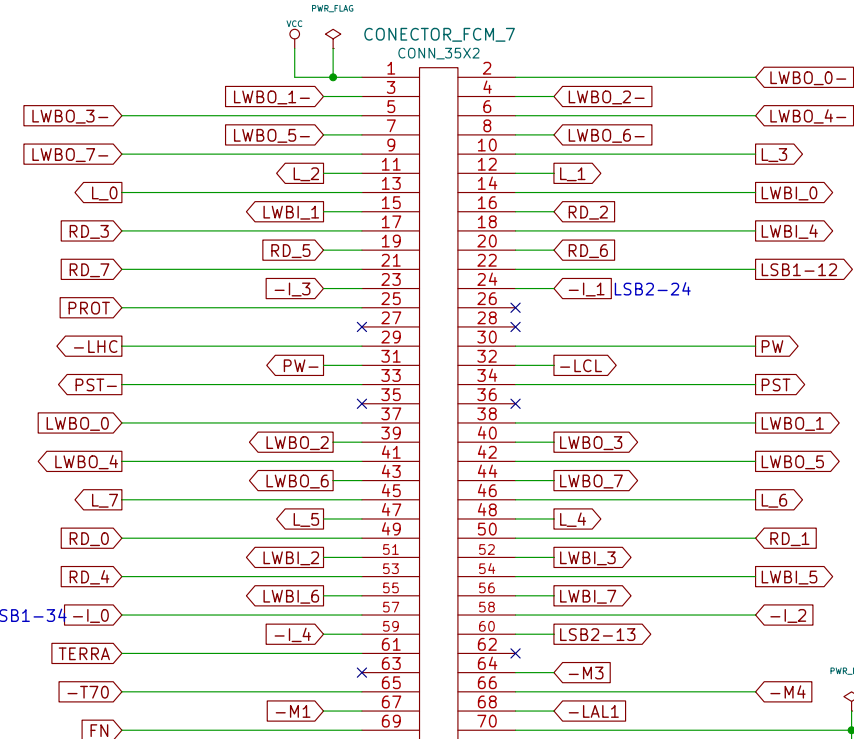
Placa FCM-7: Interface com memória
