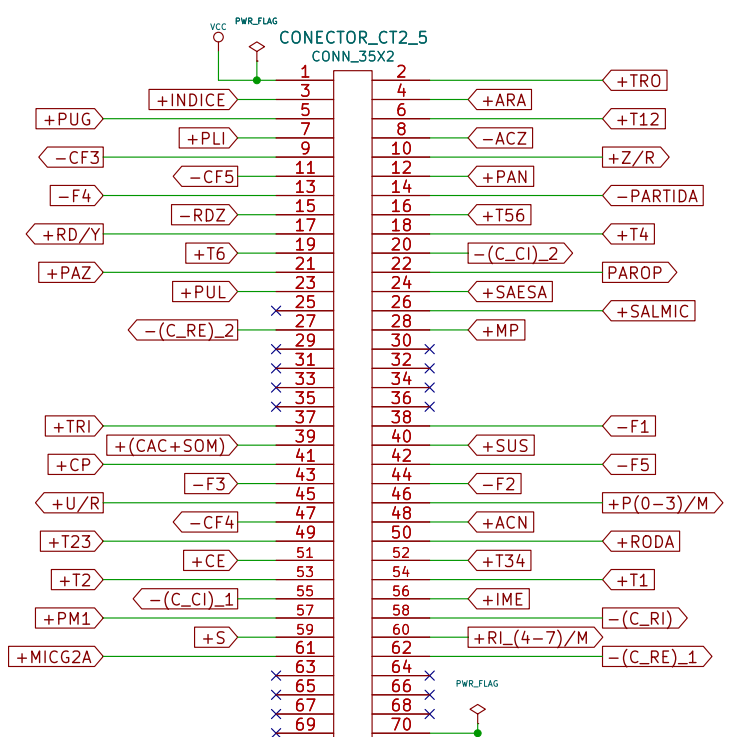
Placa CT2-5: Sinais de controle
