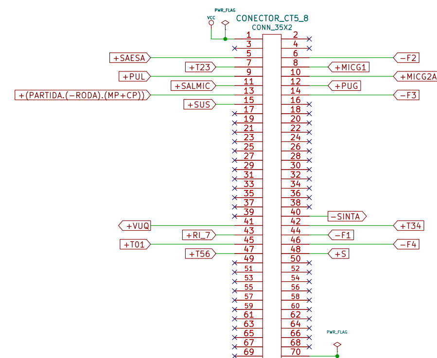
Placa CT5-8: Sinais de controle
