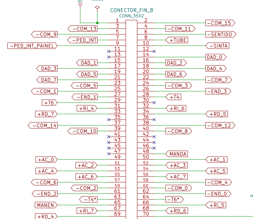
Placa FIN-8: Sinais para cartões de interface
