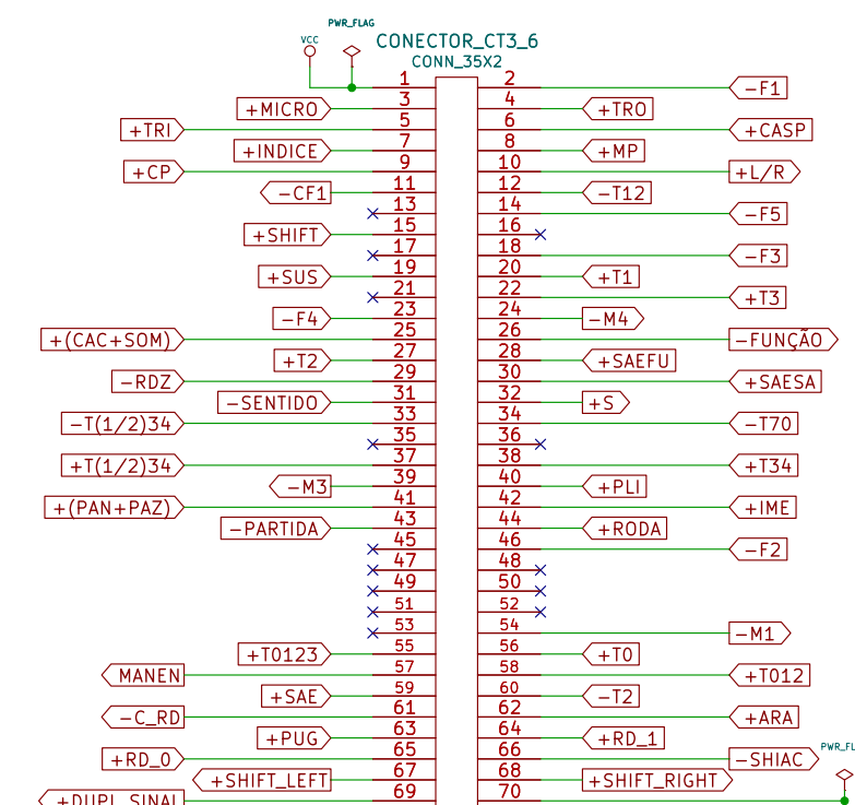
Placa CT3-6: Sinais de controle
