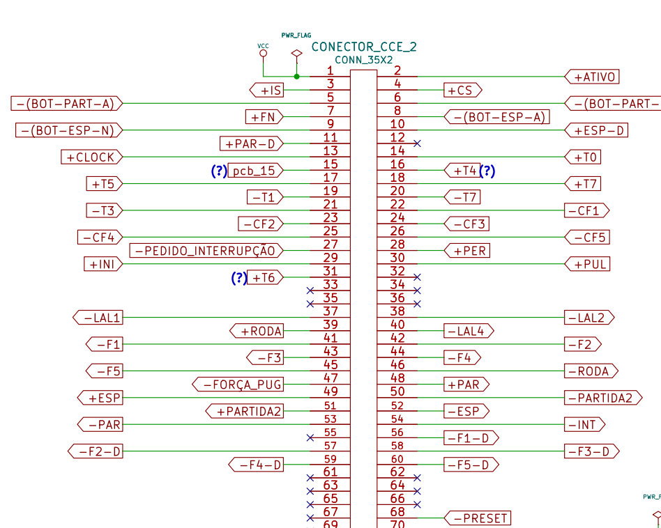
Placa CCE-2: Controle de estado.
