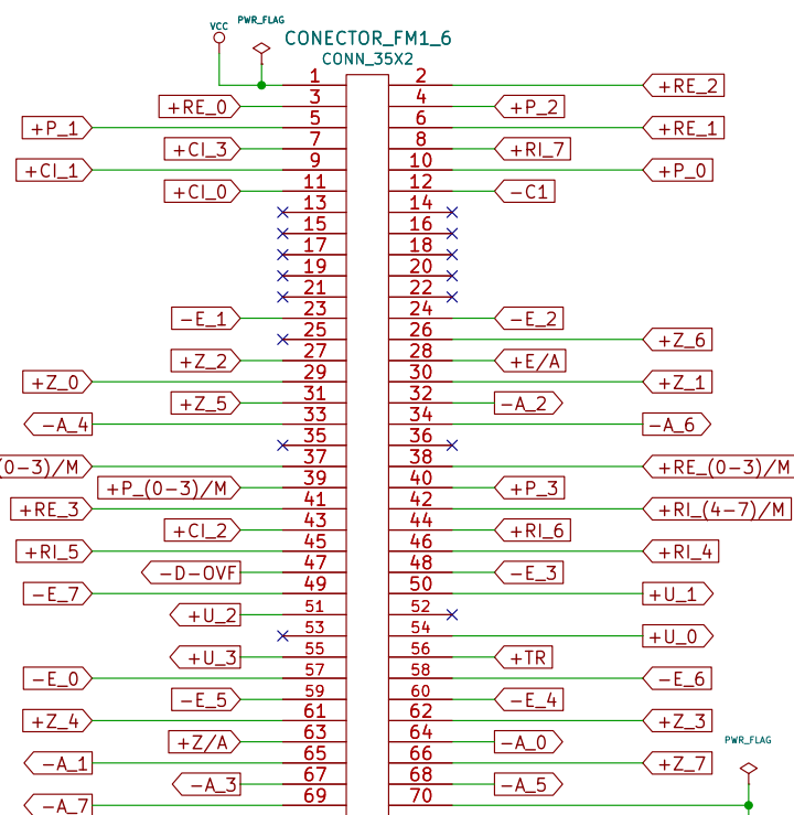
Placa FM1-6: Mais-um e porta de seleção 6
