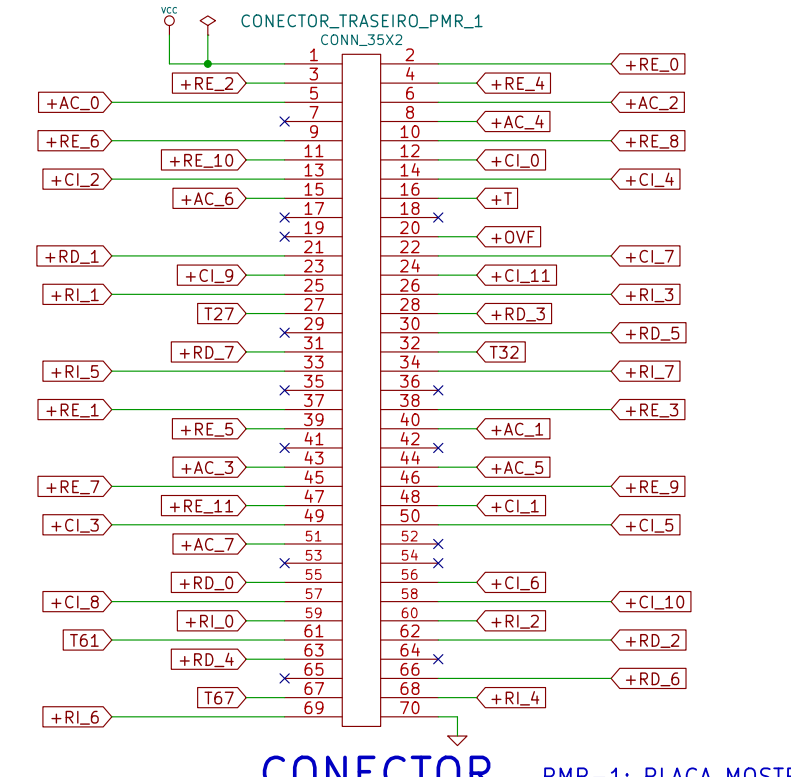
CONECTOR TRASEIRO
