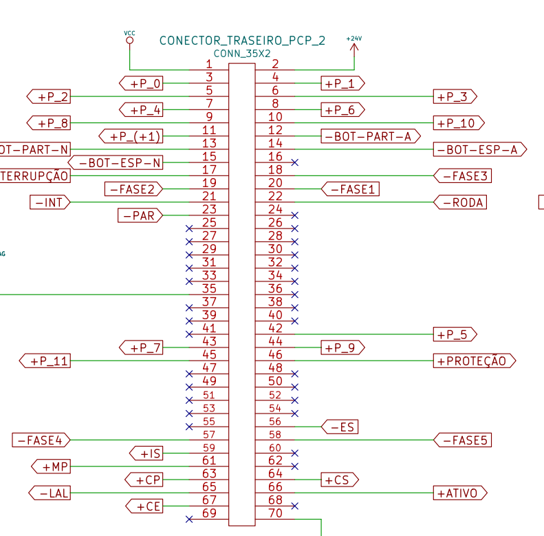
CONECTOR TRASEIRO
