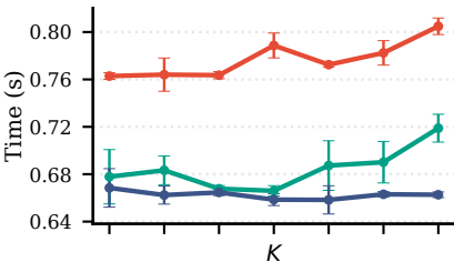
Profile: gather_all_cpu
