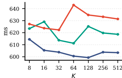
Profile: gather_all_cpu
