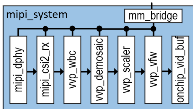
Figure 6-19 : mipi_system modules
