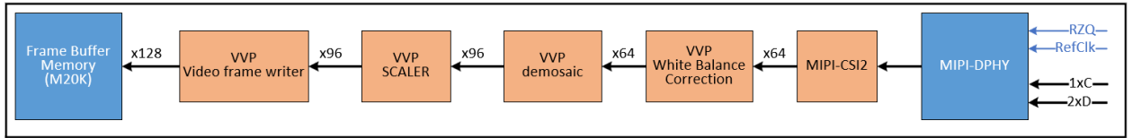
Figure 2-4 : MIPI CSI-2 Input Path
