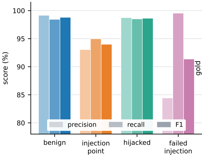
(a) Step head: precision / recall / F1 per class
