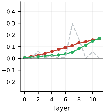
NPO (s0)
