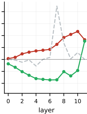
NPO (s2)
