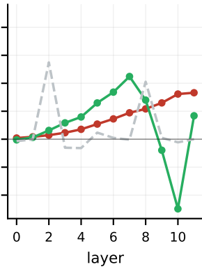
NPO (s1)
