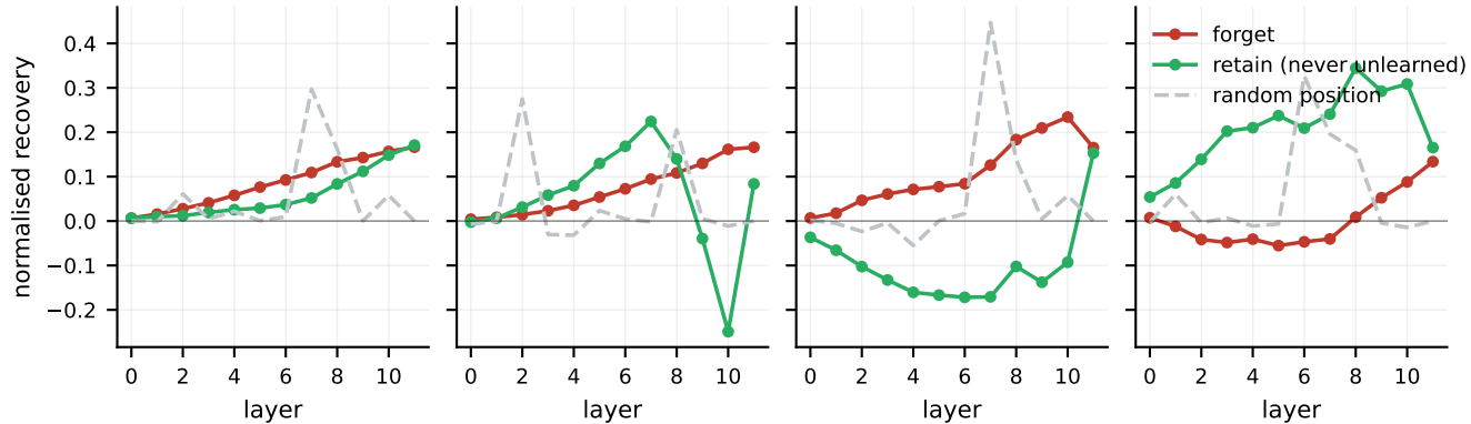
NPO (s0)
