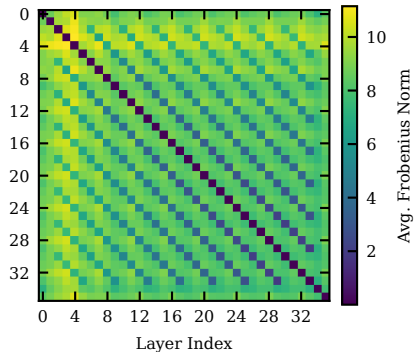
Huginn-0125
