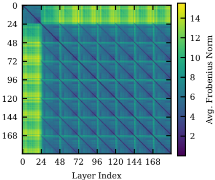
Ouro 1.4B
