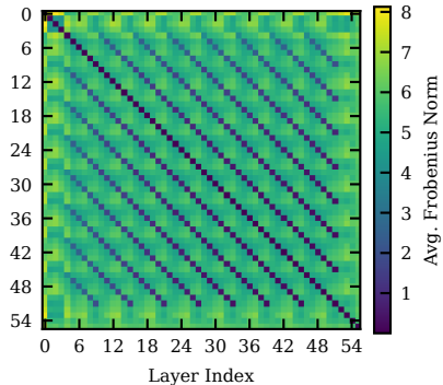
Retrofitted Llama
