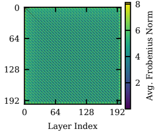
Retrofitted Llama
