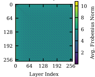
Retrofitted TinyLlama
