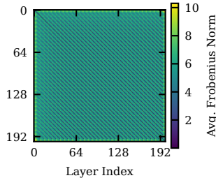
Retrofitted OLMo
