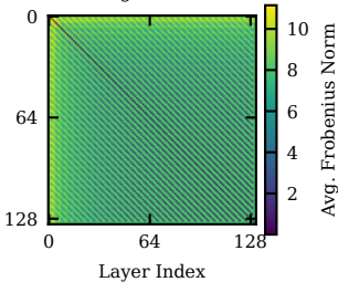
Hugginn-0125
