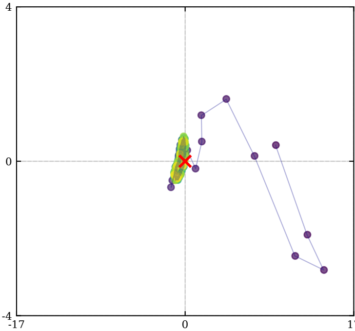
Token: " 3" L2
