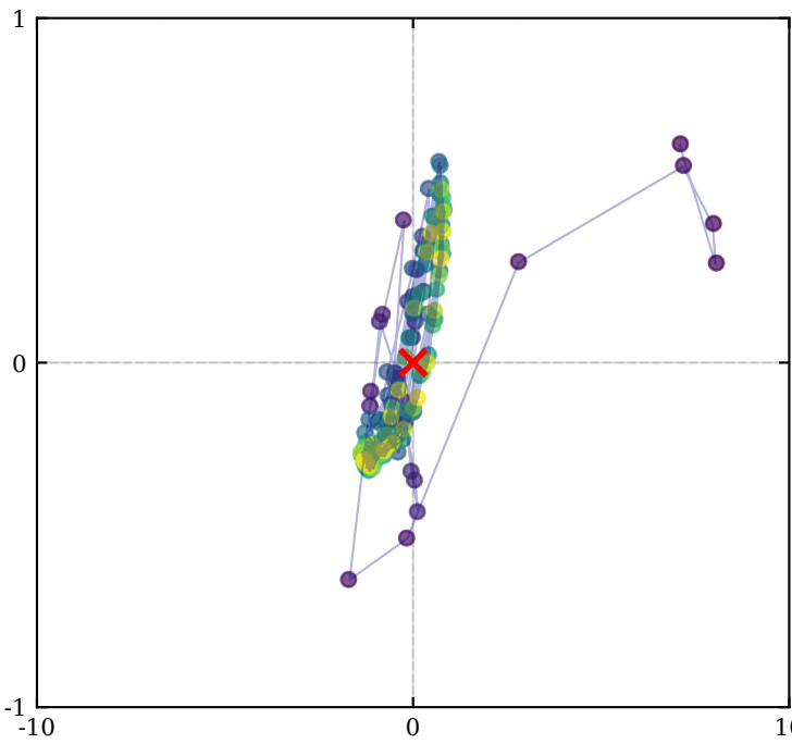
Token: " 3" L2
