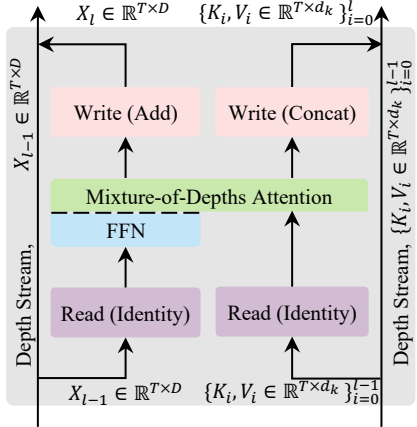
(d) Mixture-of-Depths Attention
