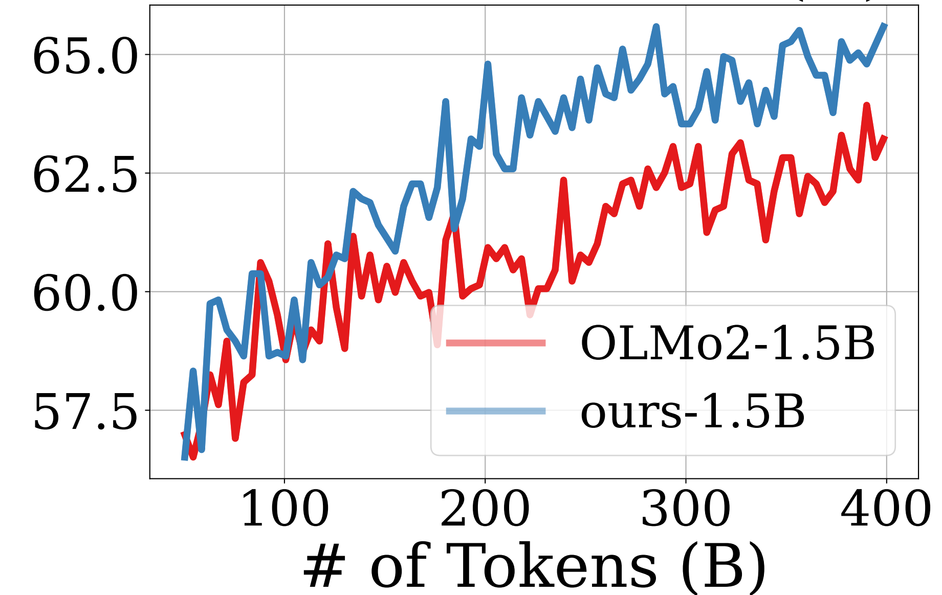
WinoGrande Acc. (%)
