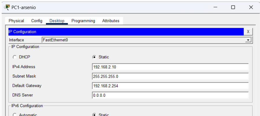
Рис. 7: Настройка IP-адреса на PC1-arsenio
