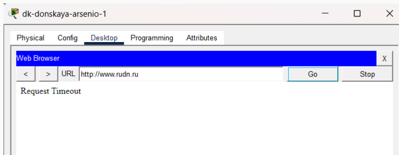
Рис. 8: Проверка ограничения доступа дисплейного класса к www.rudn.ru
