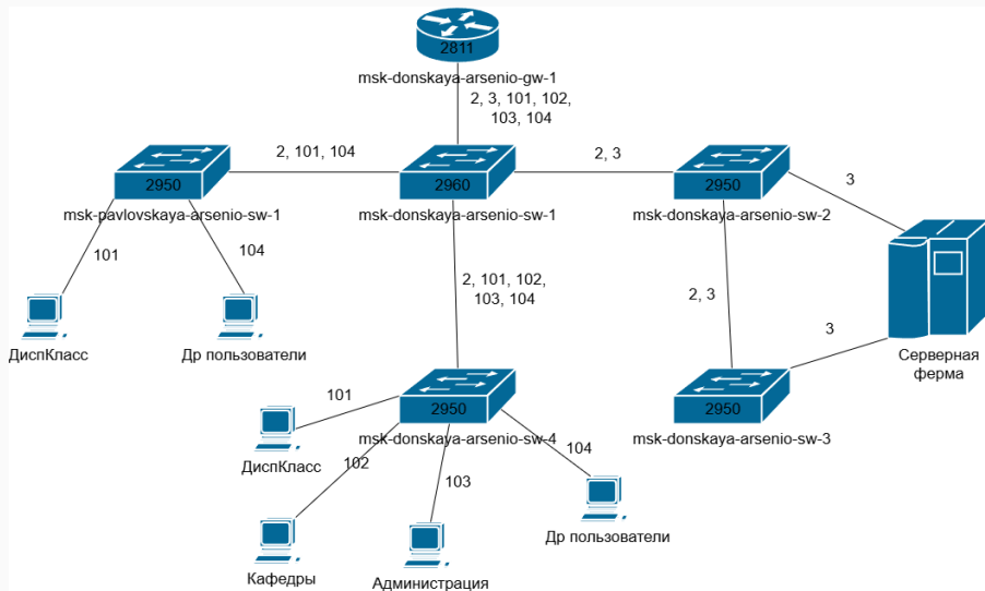
Рис. 2: Схема L2: распределение VLAN по линкам и портам
