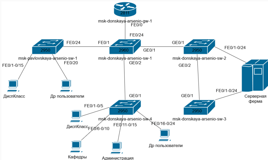
Рис. 1: Схема L1: физические соединения и интерфейсы
