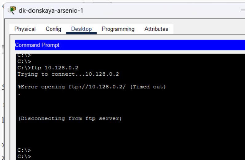
Рис. 6: Проверка запрета FTP-доступа к web-серверу для обычного пользователя
