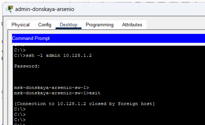
Рис. 13: Проверка SSH-доступа администратора Донской к сети управления
