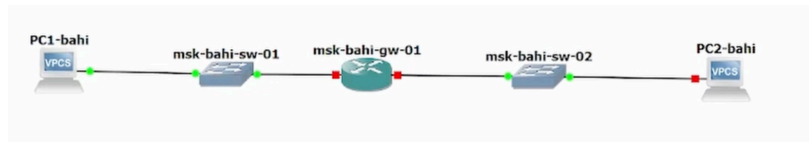
Рисунок 2.21: Топология сети в GNS3 с переименованными устройствами
