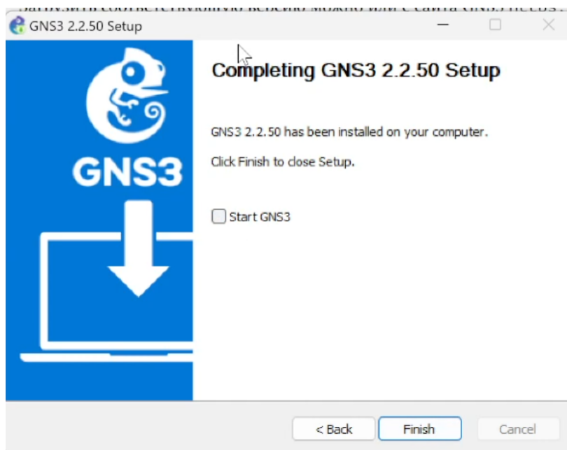
Рисунок 3.2: Завершение установки
