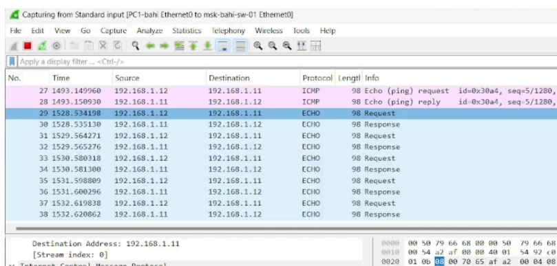
Рисунок 2.12: Полученная информация по эхо-запросу в UDP-моде к узлу PC-1
