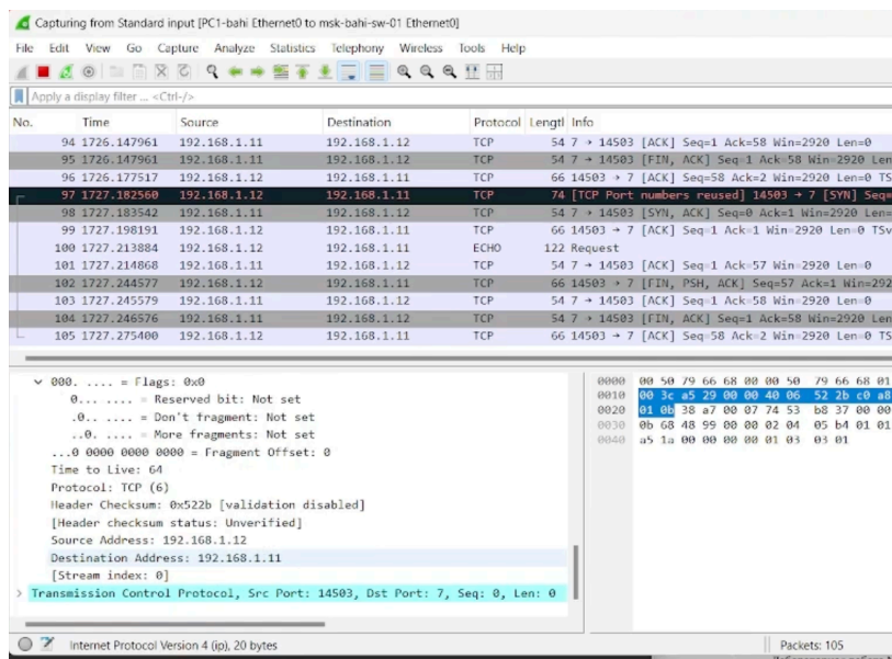
Рисунок 2.17: Полученная информация по эхо-запросу в TCP-мде к узлу PC-1
