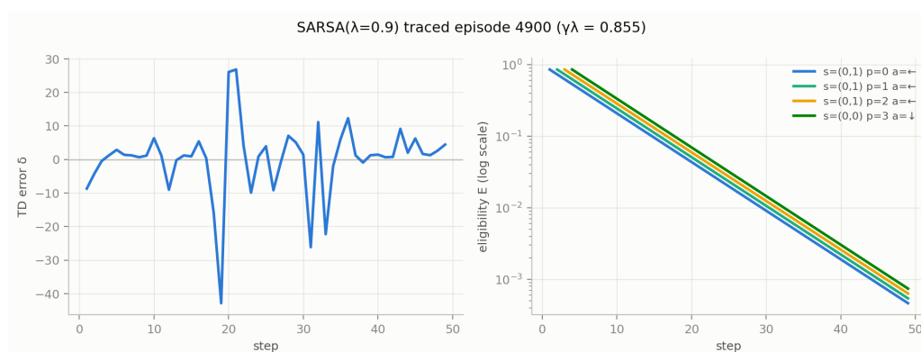
شکل ۸: خطای Temporal Difference \delta و Eligibility Traces E در اپیزود 4900
