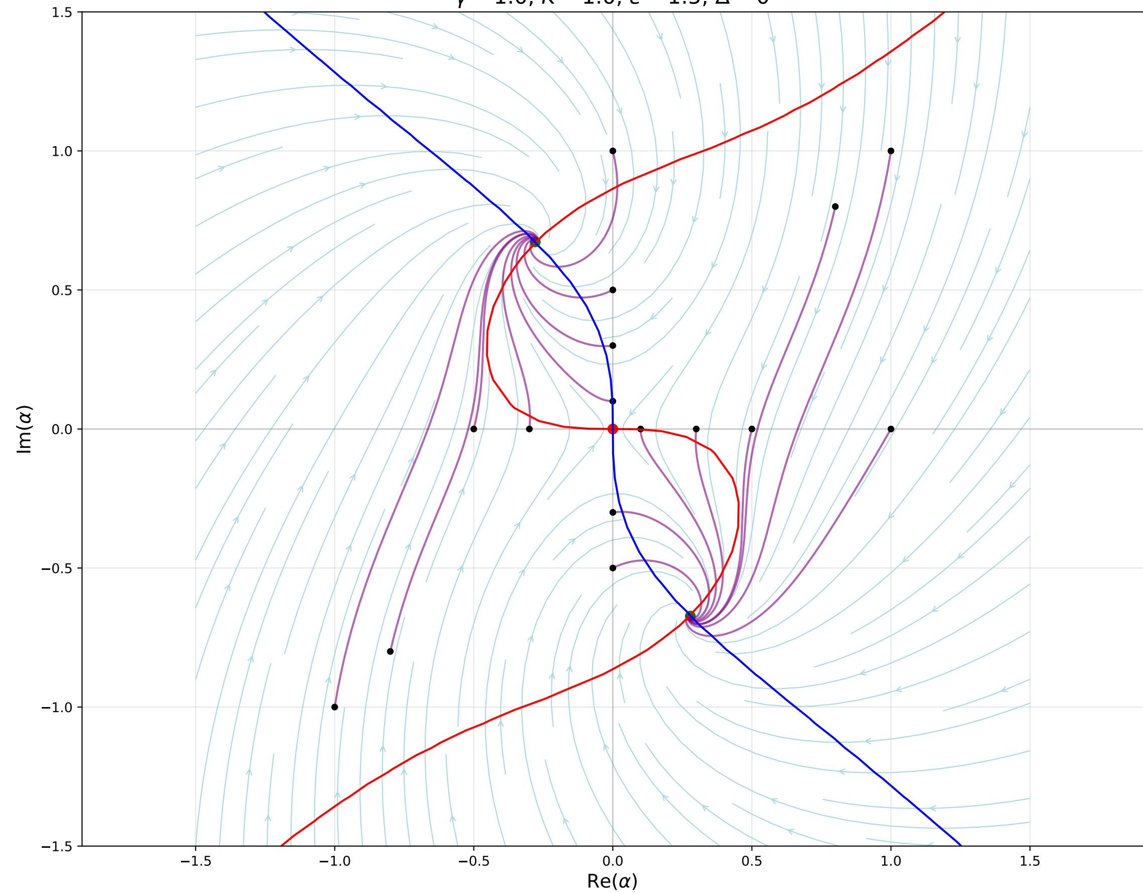
Espacio Fase: pérdida de 2 fotones \gamma = 1.0, K = 1.0, \varepsilon = 1.5, \Delta = 0
