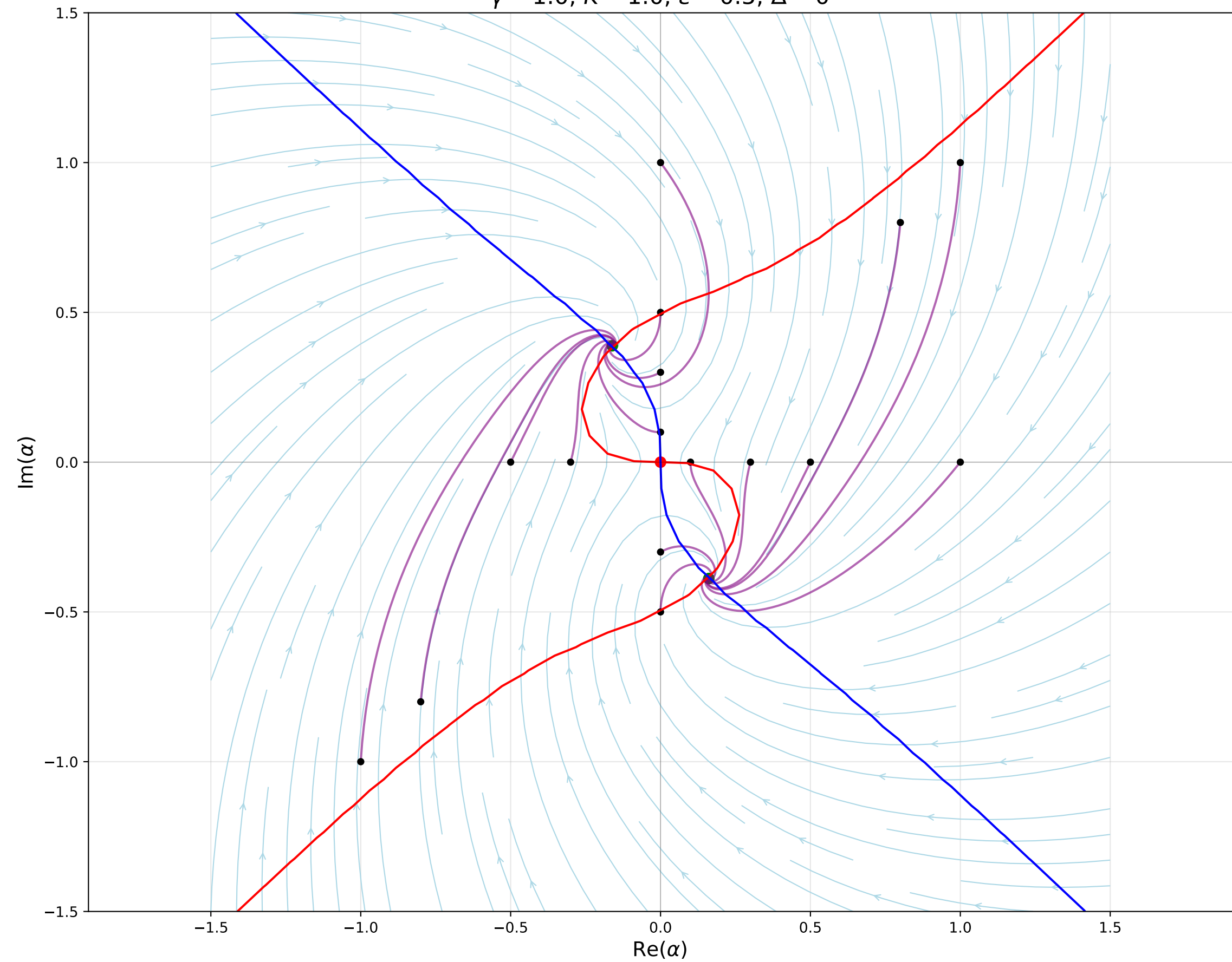
Espacio Fase: pérdida de 2 fotones \gamma = 1.0, K = 1.0, \varepsilon = 0.5, \Delta = 0
