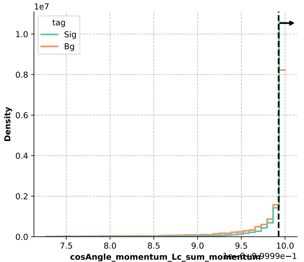
Angle_momentum_Lc_sum_momentum Distribution Angle_momentum_Lc_sum_momentum Distribution
