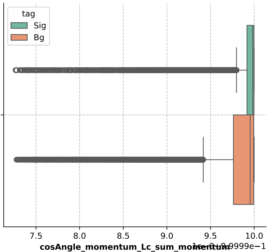
Angle_momentum_Lc_sum_momentum Distribution Angle_momentum_Lc_sum_momentum Distribution
