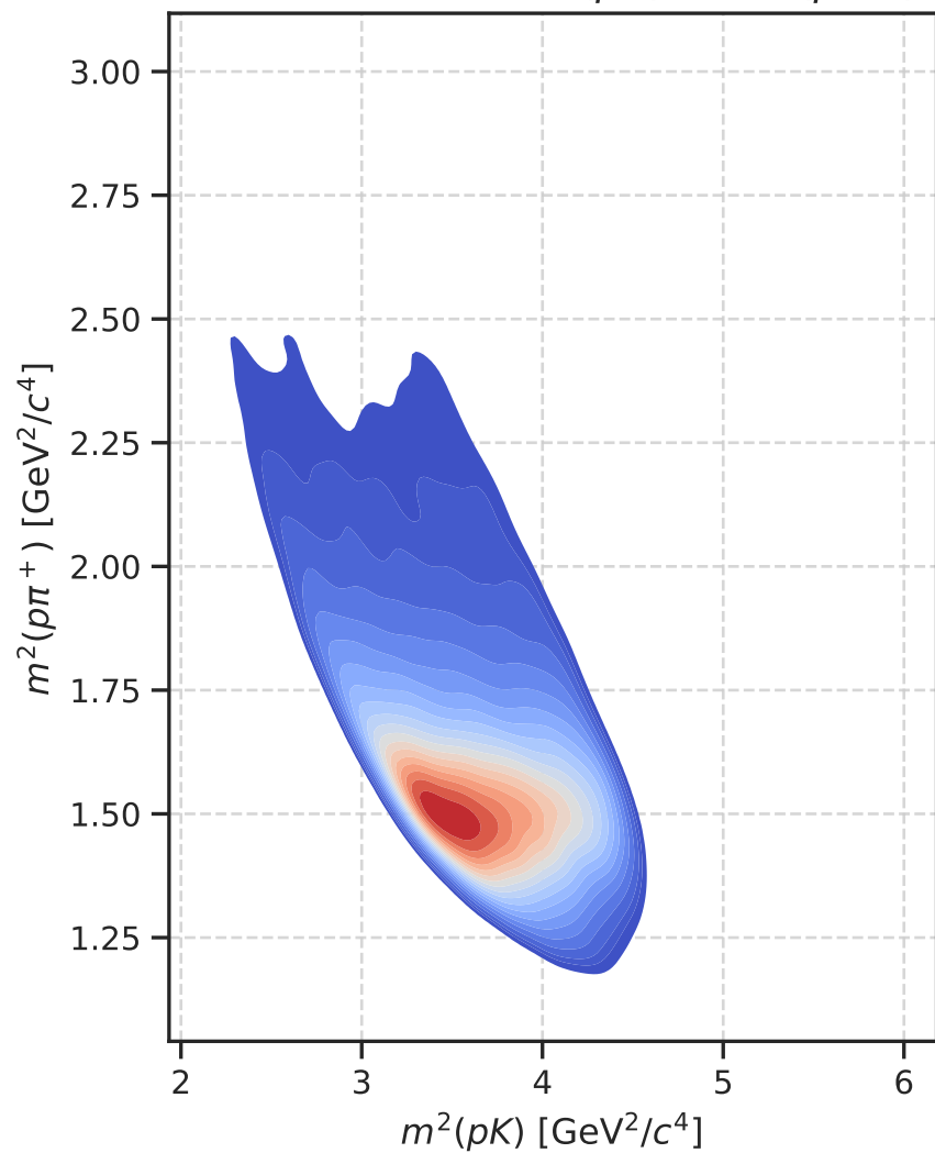
KDE Dalitz Plot: m^2(pK) vs m^2(p\pi^+)
