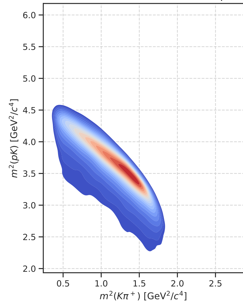
KDE Dalitz Plot: m^2(K\pi^+) vs m^2(pK)
