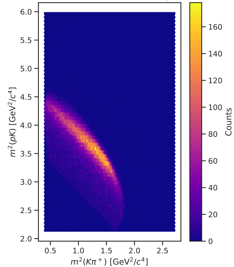
Dalitz Plot: m^2(K\pi^+) vs m^2(pK)
