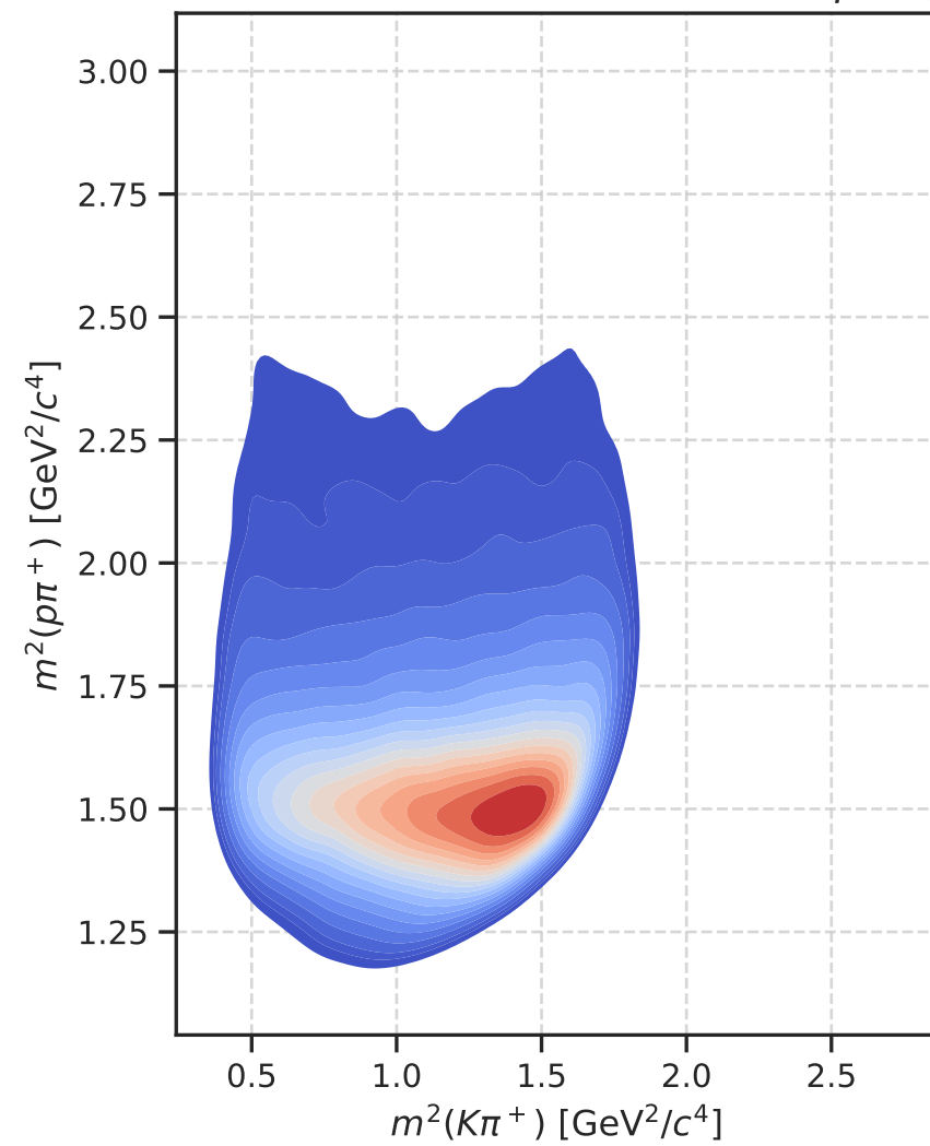
KDE Dalitz Plot: m^2(K\pi^+) vs m^2(p\pi^+)
