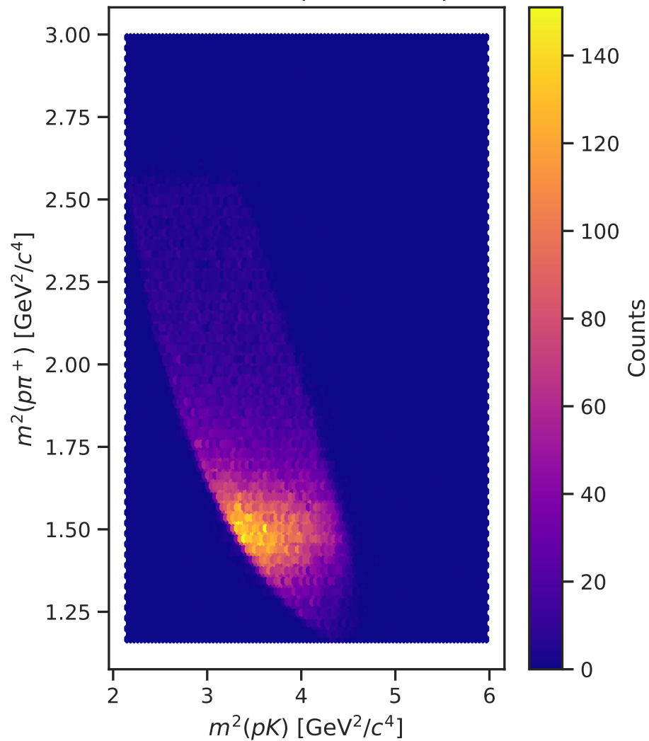
Dalitz Plot: m^2(pK) vs m^2(p\pi^+)
