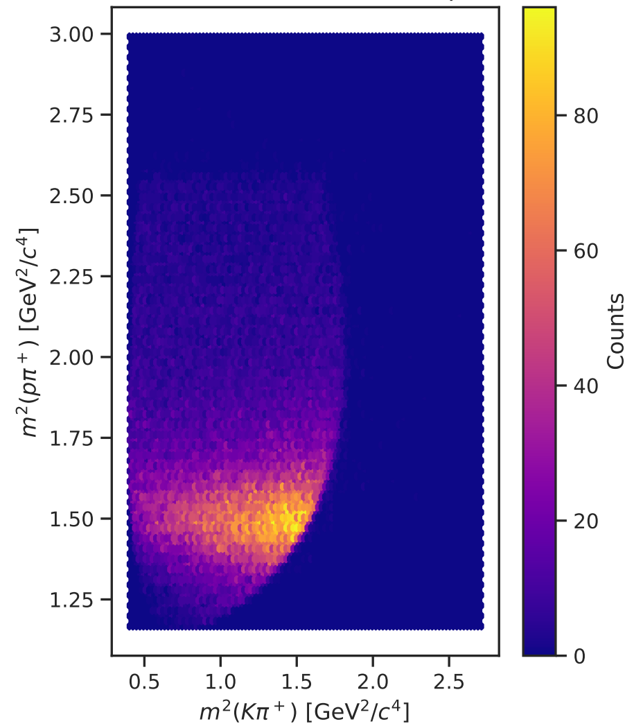
Dalitz Plot: m^2(K\pi^+) vs m^2(p\pi^+)
