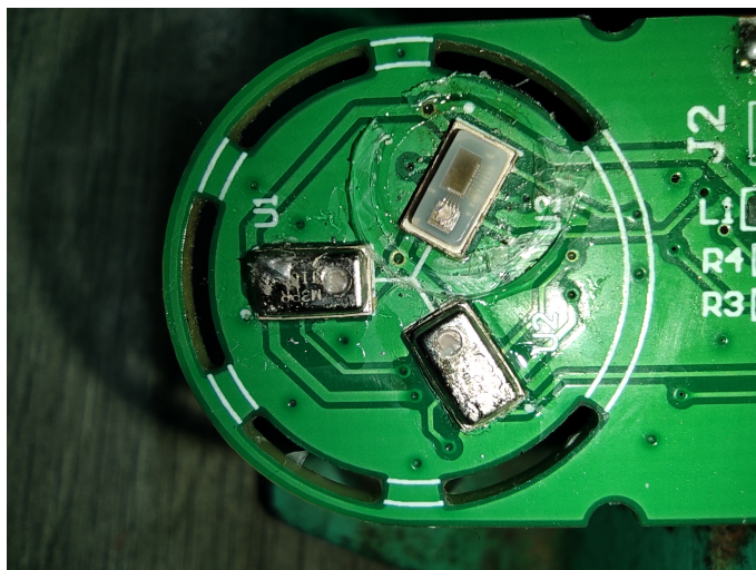
شکل ۱۵.۲: حسگر سه‌تایی ساخته شده، پس از دستکاری مکانیکی بارومترها. محفظه‌ی فلزی یکی از حسگرها به طور کامل برداشته شده.
