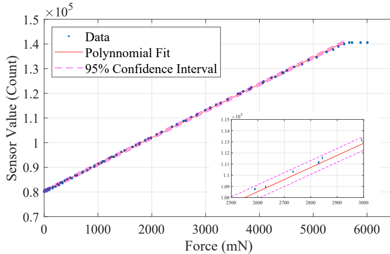
شکل ۹.۲: مدل برازش شده بر داده های حسگر.
