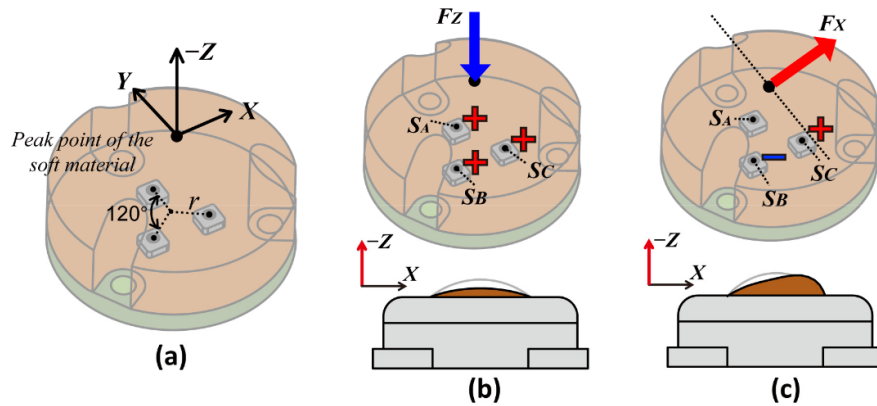
شکل ۲.۱۳: تغییرات هر کدام از حسگرها در حضور نیرو عمودی و مماسی [۶۱].
