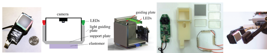
شکل ۸.۱: ساختار حسگر لامسه Gelsight معرفی شده در [۴۵].
