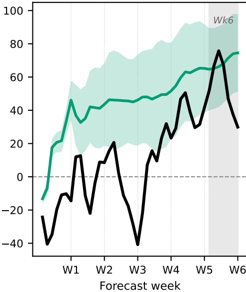
ECMWF
