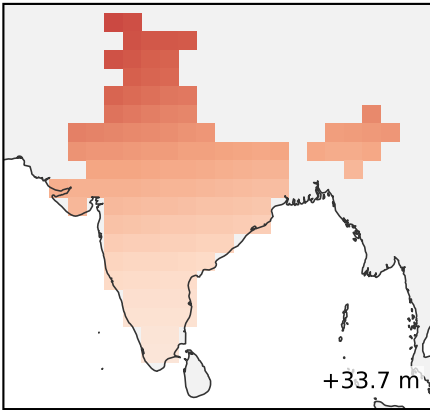
ECMWF
