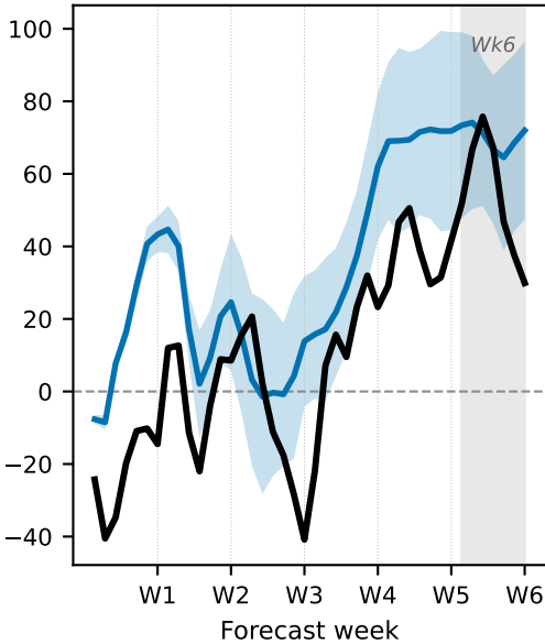
FuXi-S2S
