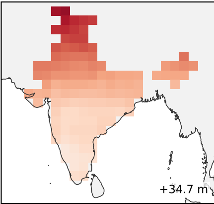
FuXi-S2S
