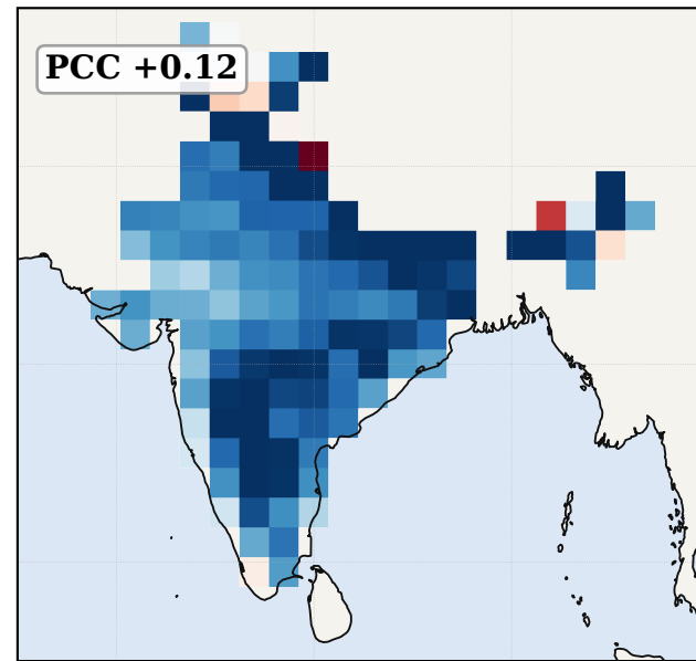
FuXi-S2S
