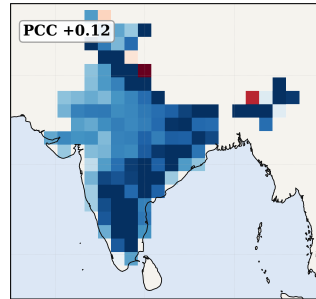
ECMWF
