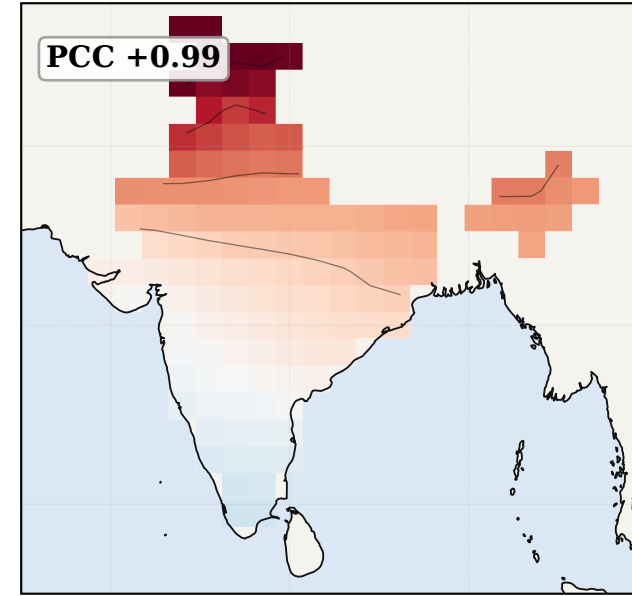
ECMWF
