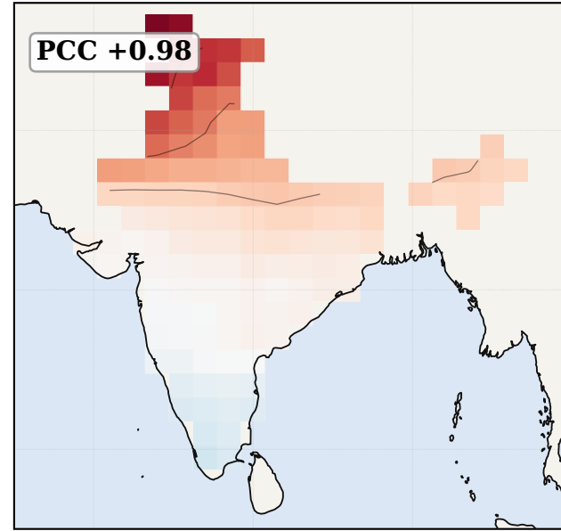
FuXi-S2S
