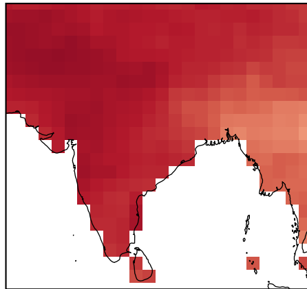
FuXi
