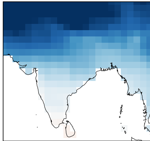
FuXi
