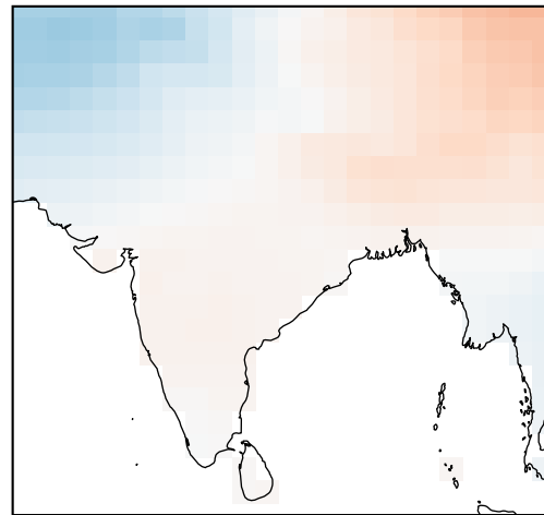
ECMWF
