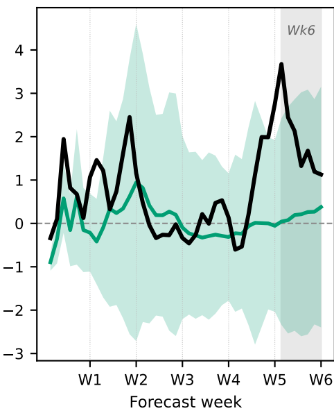
ECMWF
