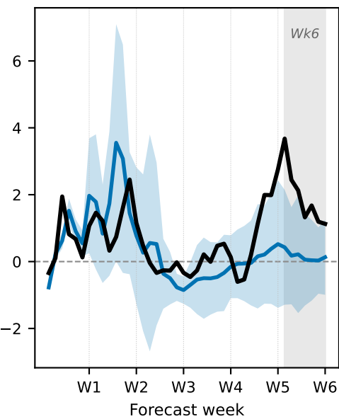
FuXi-S2S
